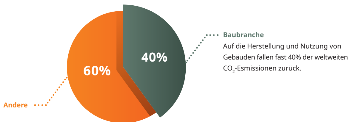
Weltweite Kohlenstoffemissionen
